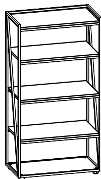
LMMC 80 800x430x1517
