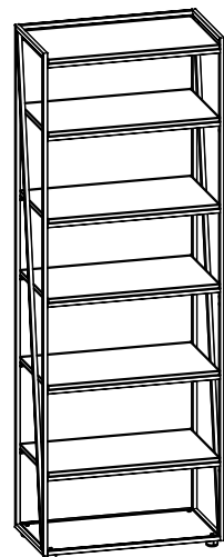
LMHC 80 800x430x2253
